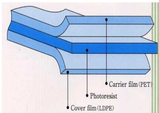
（干膜光刻胶结构示意图）
