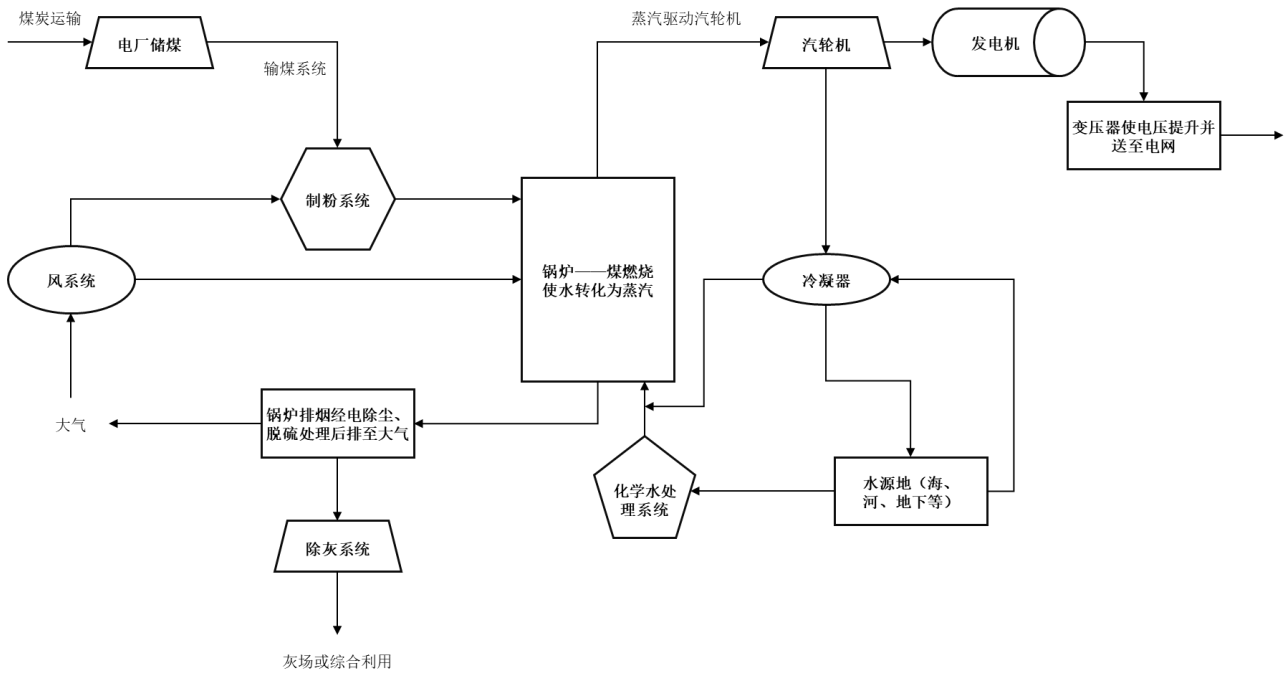
图：火电发电/热电联产流程图
