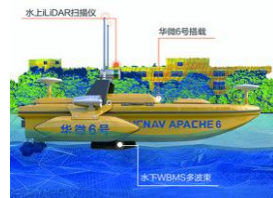
水上水下无人化点云数据采集方案
