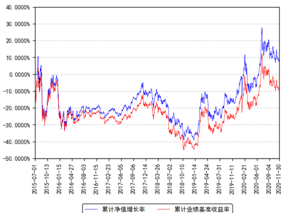
南方中证互联网指数分级累计净值增长率与同期业绩比较基准收益率的历史走势对比图
