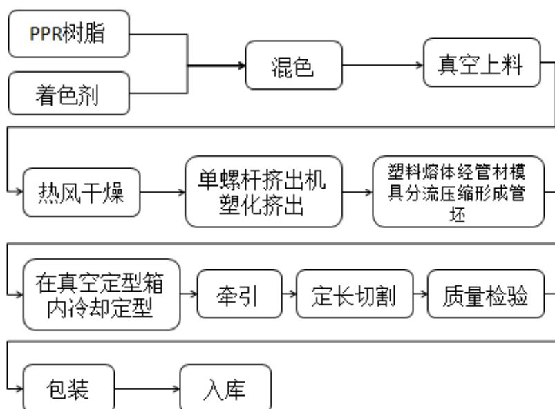
D.PPR 管材挤出成型工艺流程图
