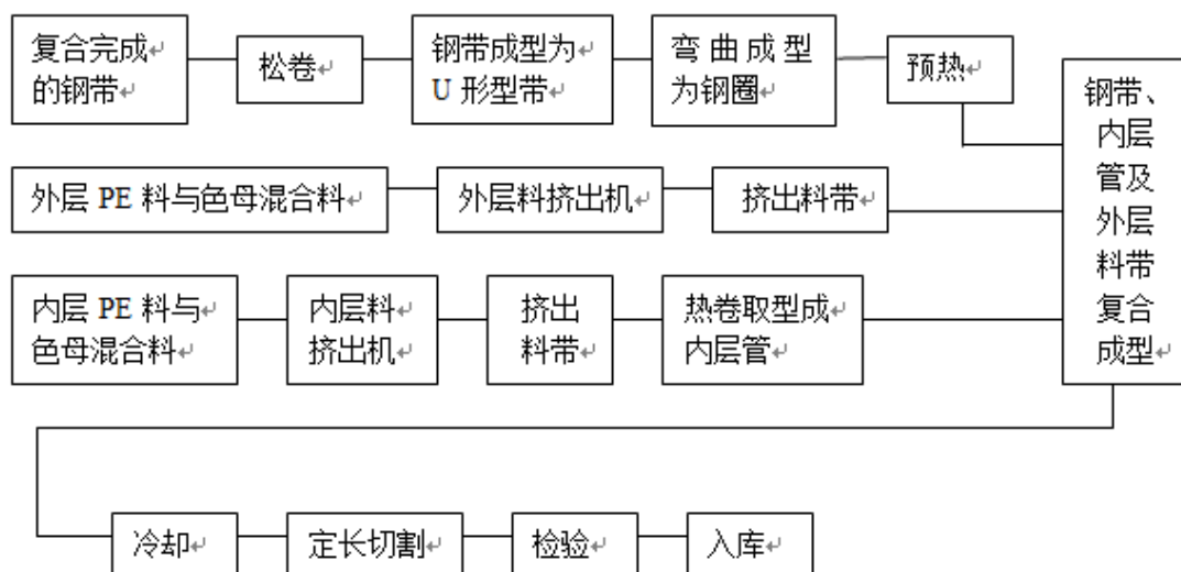
I.HDPE 中空壁缠绕管成型工艺流程图
