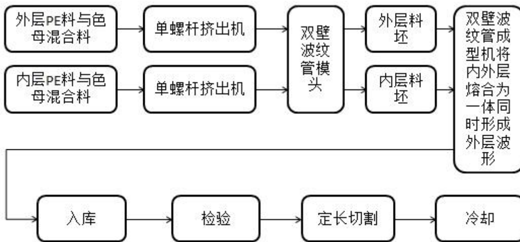
B.PE 双壁波纹管成型工艺流程图
