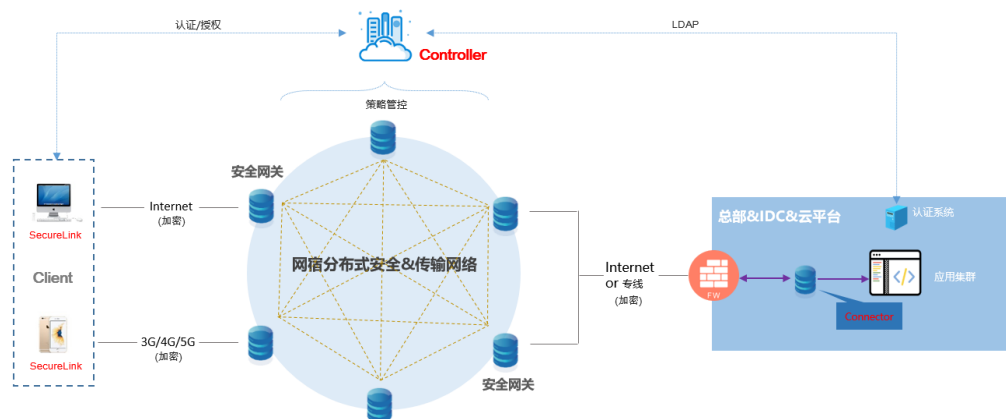
网宿 SecureLink 产品架构
