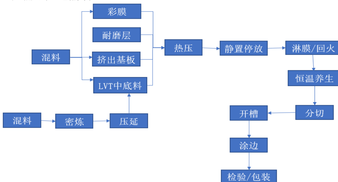
(3) AB贴合热压生产工艺流程图
