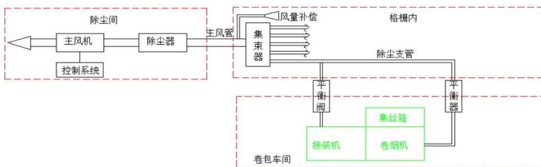
集中工艺风力除尘系统流程图
