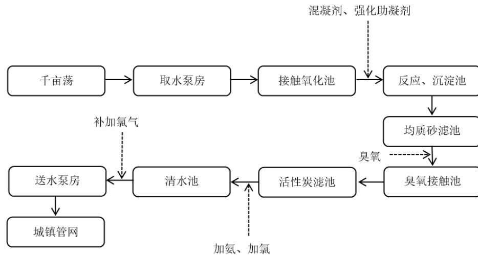
自来水工艺流程图
