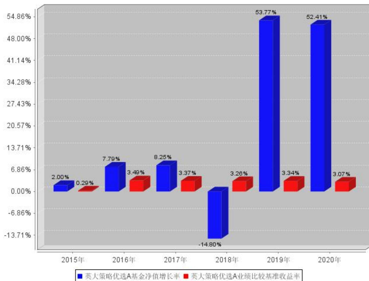
英大策略优选A自基金合同生效以来基金每年净值增长率及其与同期业绩比较基准收益率的对比图
