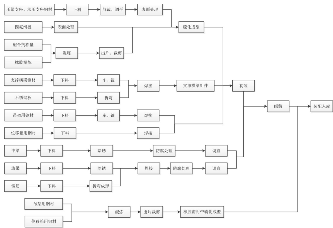
5、模数式桥梁伸缩装置生产工艺流程图
