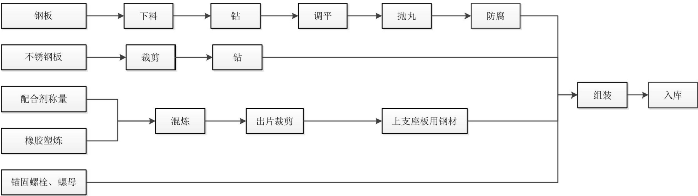
6、梳齿板式桥梁伸缩装置生产工艺流程图
