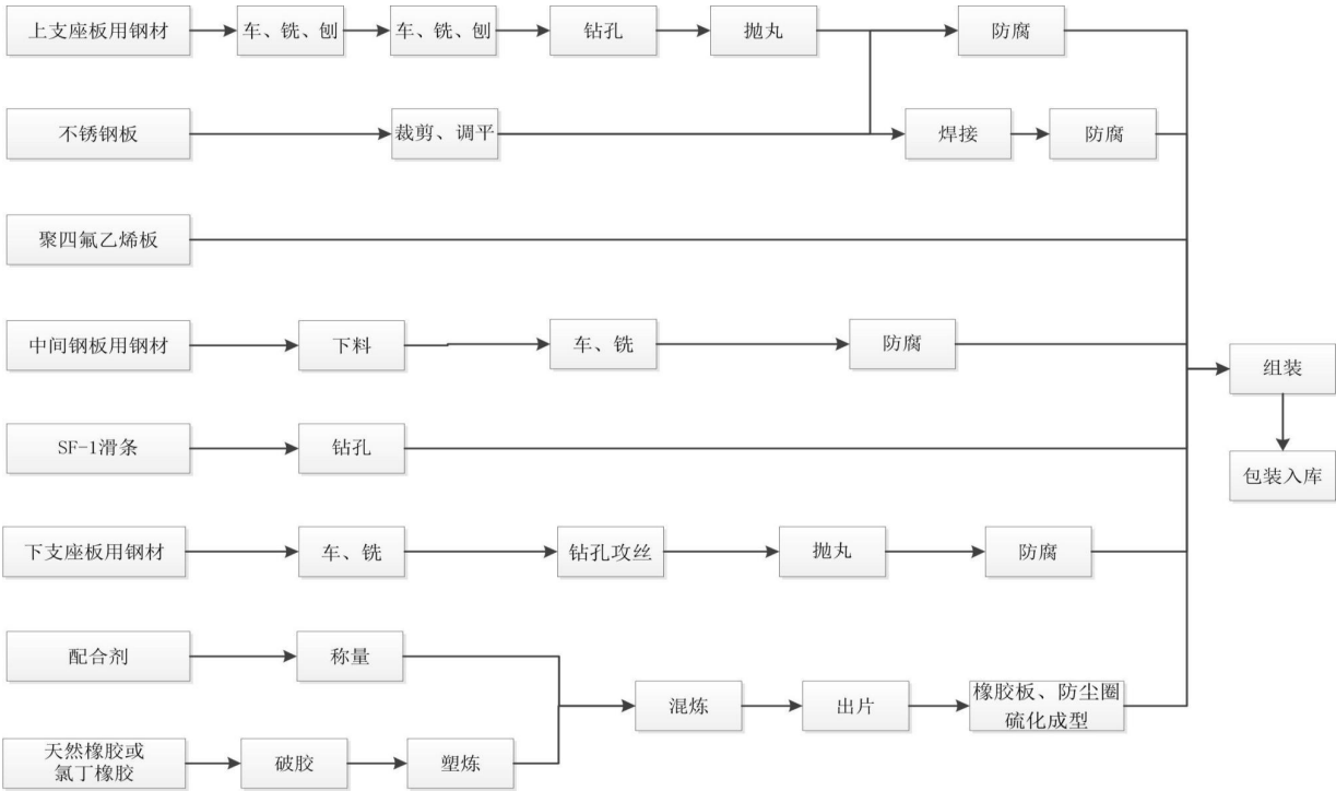
2、盆式支座工艺流程图
