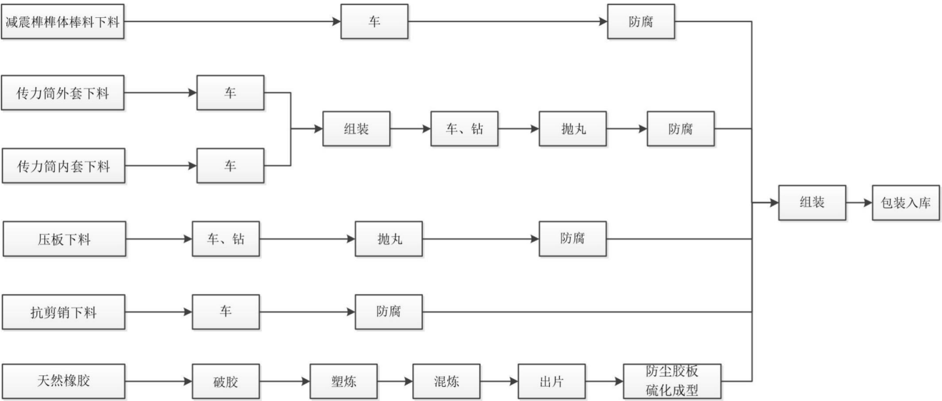
7、防落梁装置工艺流程图
