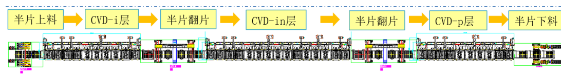
I-IN-P 三段镀膜在线多腔室 PECVD 量产设备布局
