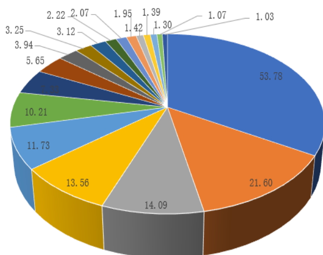
2020年欧洲市场主要地区光伏累计装机容量 (单位: GW)
