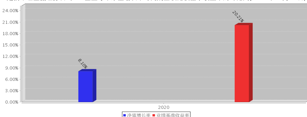
建信中证全指证券公司ETF基金每年净值增长率与同期业绩比较基准收益率的对比图(2020年12月31日)
