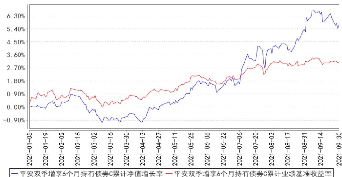
平安双季增享6个月持有债券C累计净值增长率与同期业绩比较基准收益率的历史走势图
