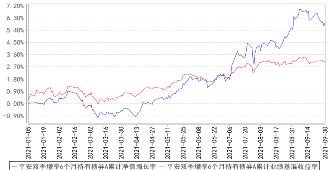
平安双季增享6个月持有债券A累计净值增长率与同期业绩比较基准收益率的历史走势图
