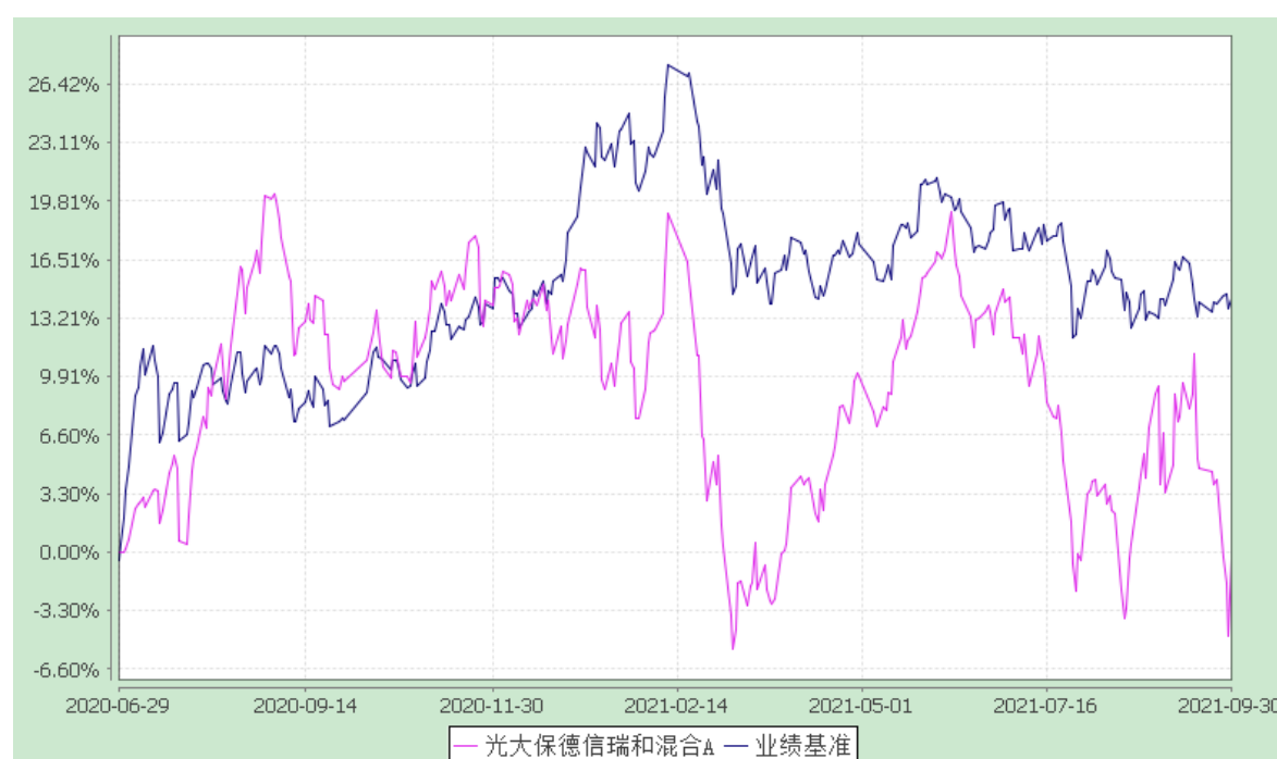
光大保德信瑞和混合型证券投资基金 累计净值增长率与业绩比较基准收益率的历史走势对比图 (2020 年 6 月 29 日至 2021 年 9 月 30 日)
