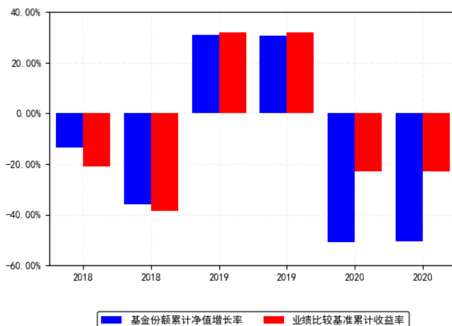
南方原油C每年净值增长率与同期业绩比较基准收益率的对比图（2020年12月31日）
