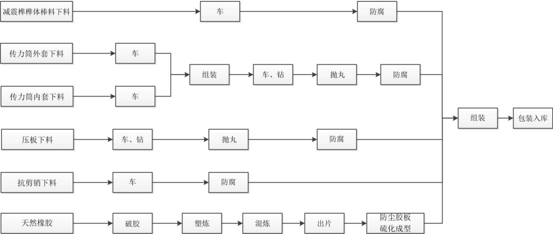
7、防落梁装置工艺流程图
