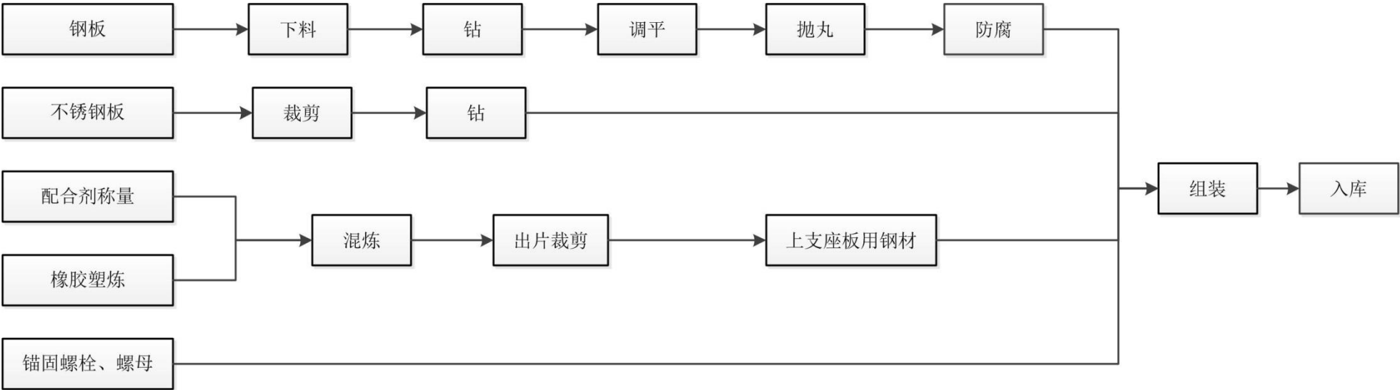
6、梳齿板式桥梁伸缩装置生产工艺流程图
