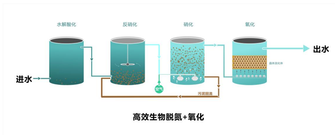
技术工艺流程图
