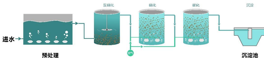
技术工艺流程图
