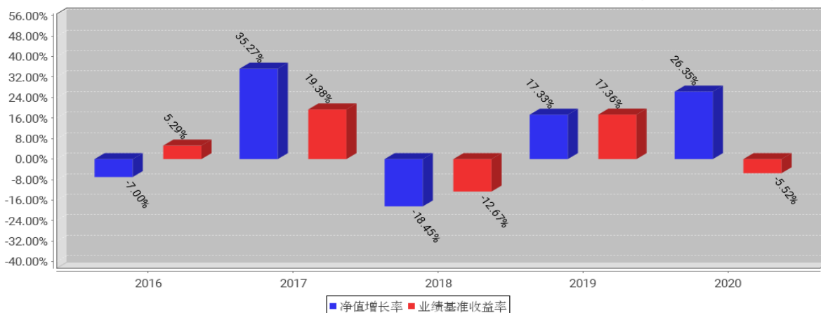
工银沪港深股票A基金每年净值增长率与同期业绩比较基准收益率的对比图(2020年12月31日)
