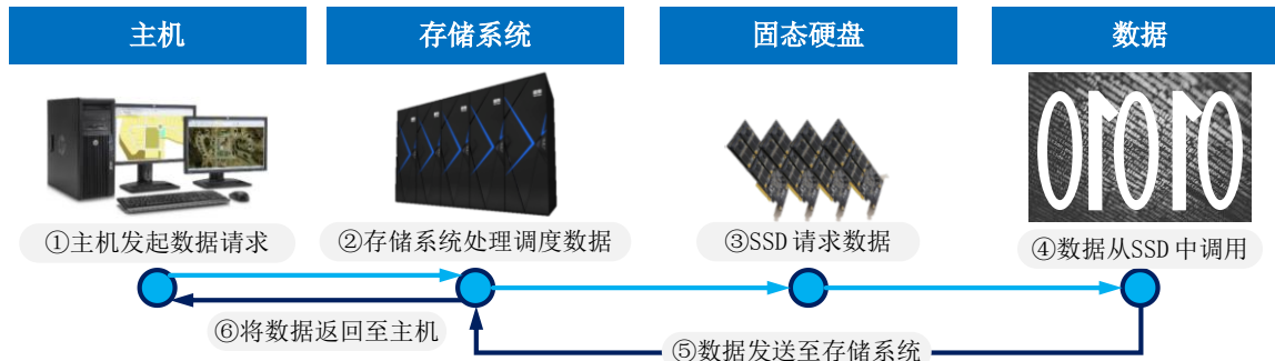
IT 系统数据读取过程
