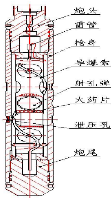
公司复合射孔器结构图
