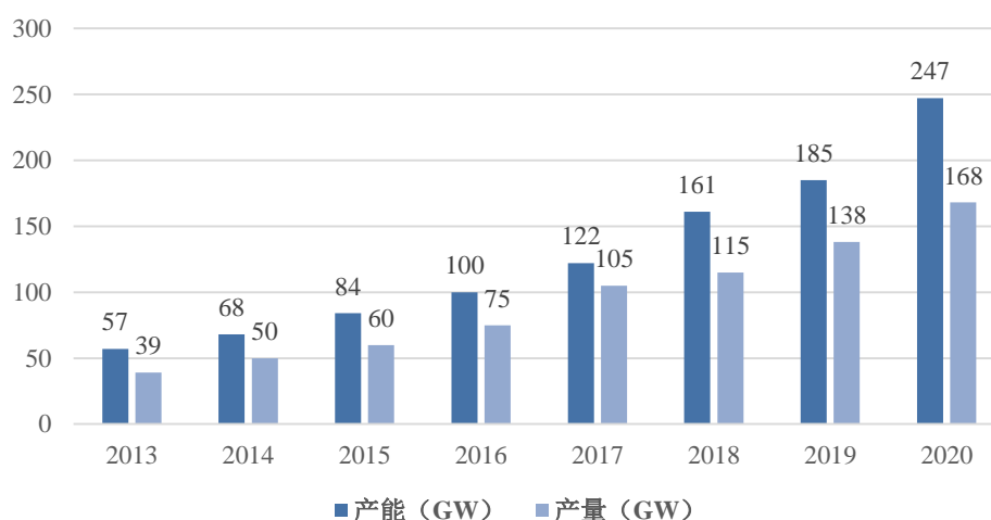
全球光伏硅片产能及产量
