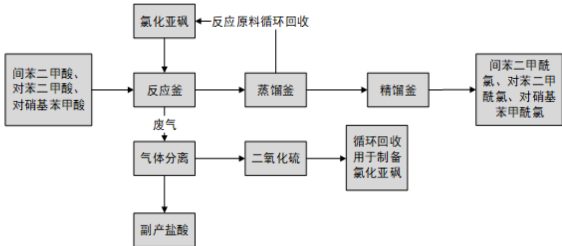
2) 间/对苯二甲酰氯、对硝基苯甲酰氯产品工艺流程简图
