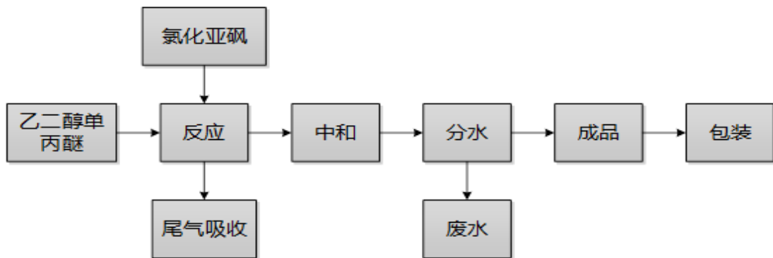
4) 聚醚酮酮产品工艺流程图
