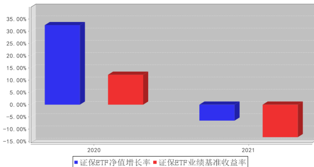
证保ETF基金每年净值增长率与同期业绩比较基准收益率的对比图
