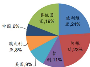
2020 年锂资源量结构
