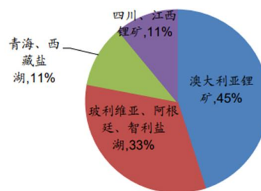
2021 年锂供给结构
