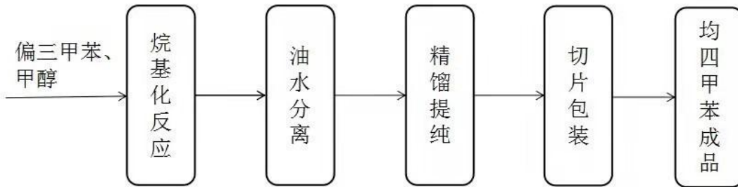
(5) 均四甲苯的工艺流程图
