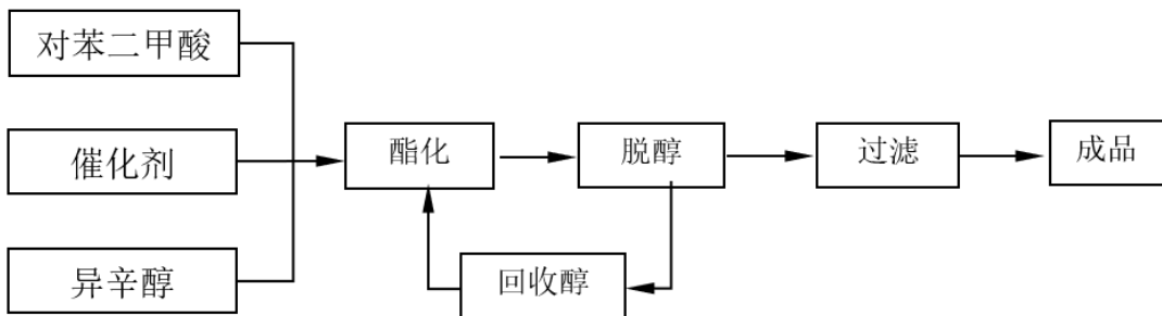
(4) 乙烯基甲苯的工艺流程图
