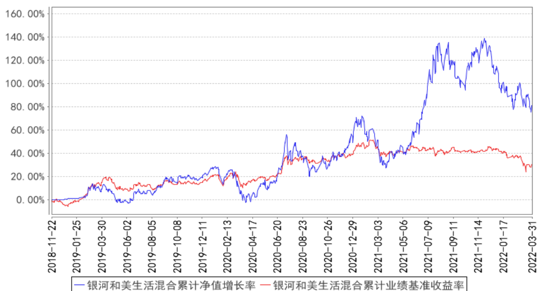
银河和美生活混合累计净值增长率与同期业绩比较基准收益率的历史走势对比图
