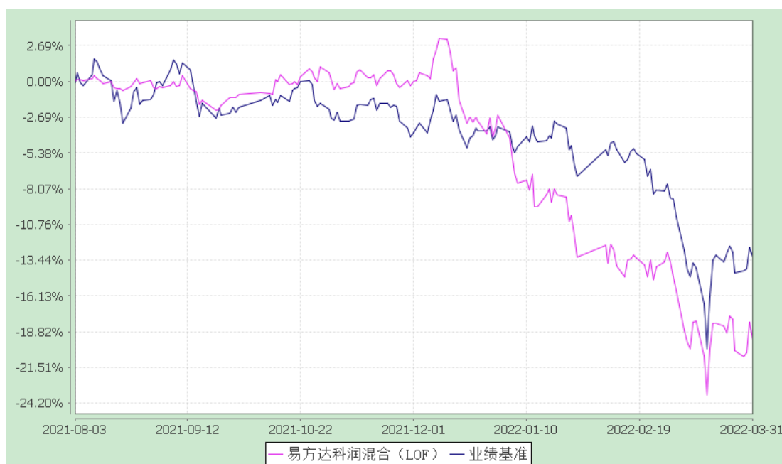
易方达科润混合型证券投资基金（LOF） 累计净值增长率与业绩比较基准收益率的历史走势对比图 （2021 年 8 月 3 日至 2022 年 3 月 31 日）
