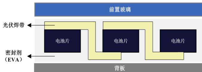
光伏焊带工作原理
