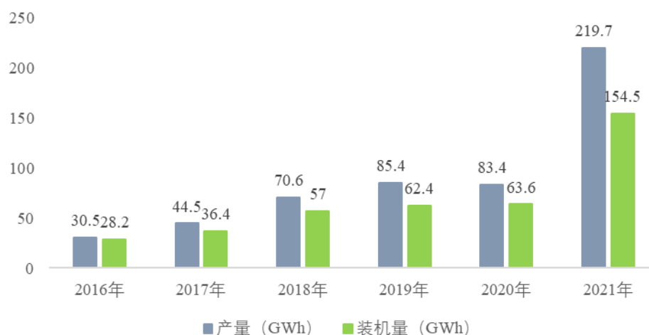
2016-2021年我国动力电池装机量和产量
