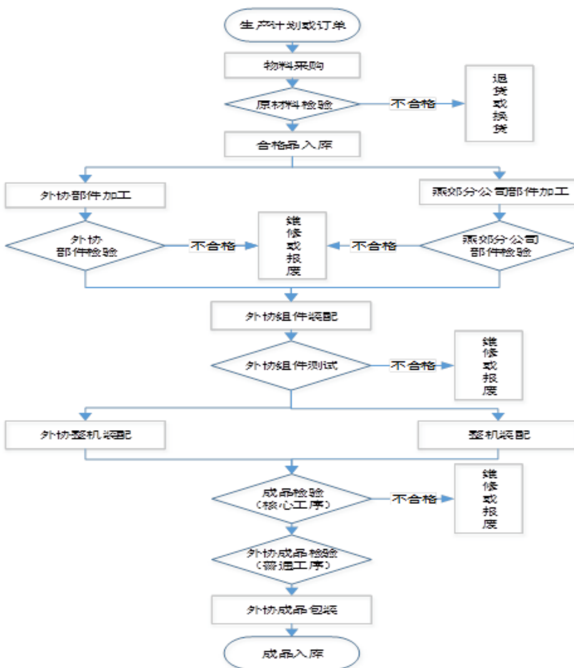
OBU 产品工艺流程
