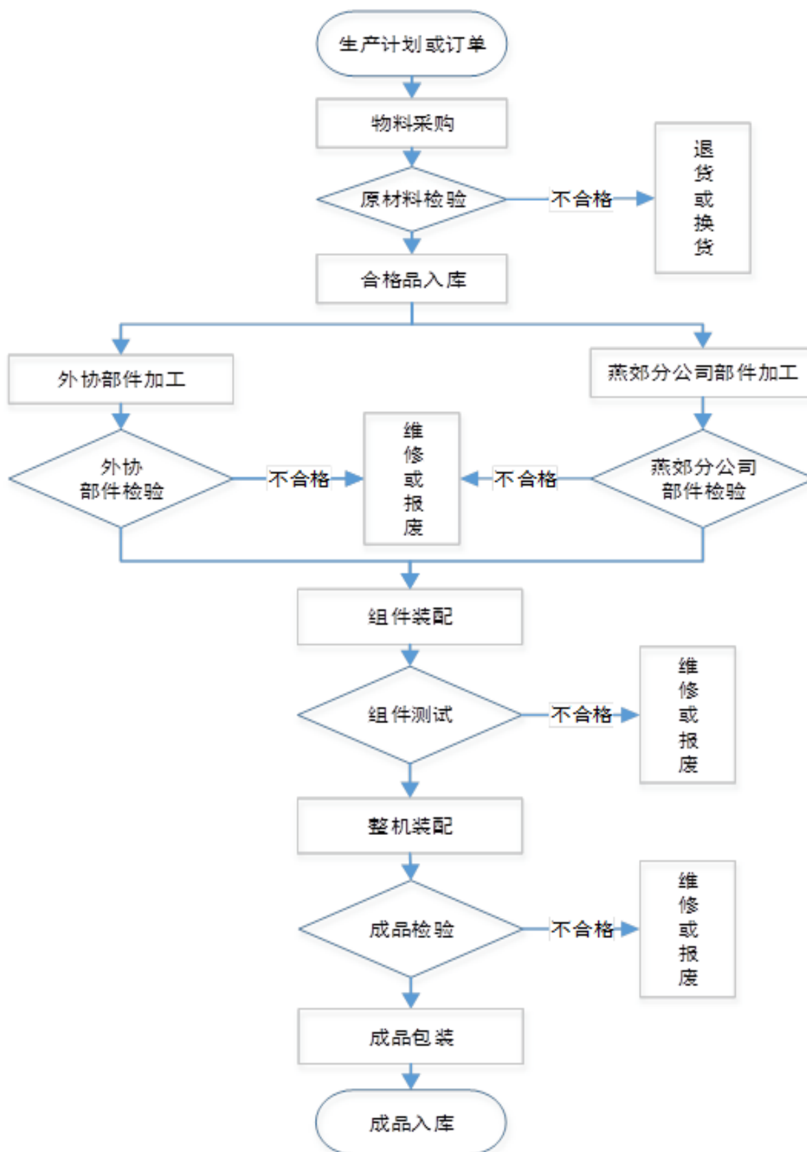
RSU、车载产品工艺流程
