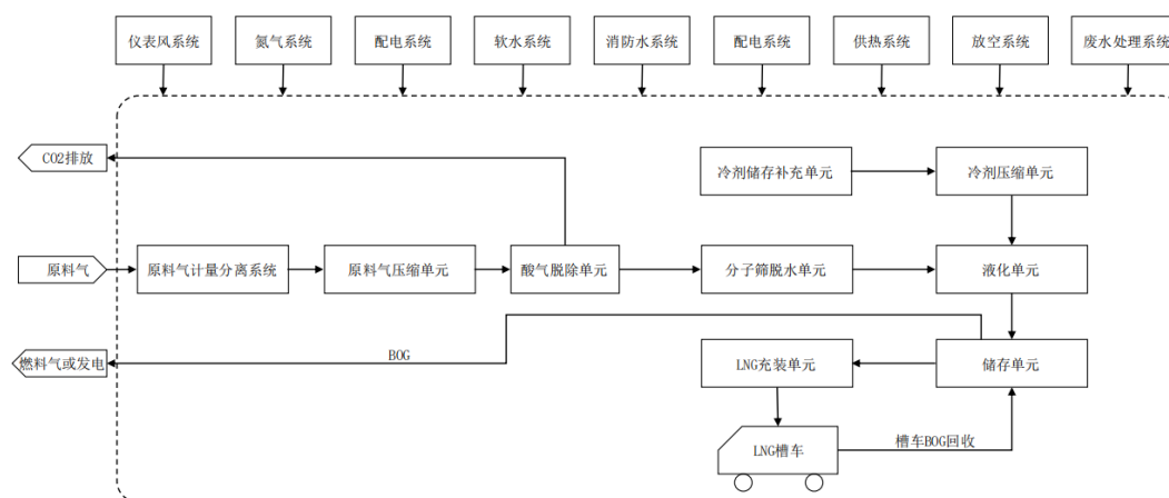
(4) 内蒙森泰 LNG 工厂工艺介绍及工艺流程图
