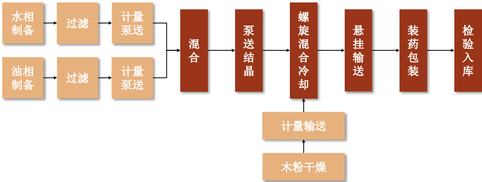
(3) 膨化硝铵炸药生产工艺流程图
