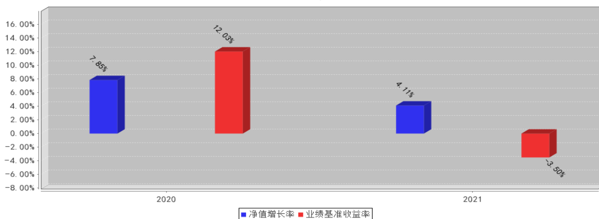
民生加银新兴产业混合A基金每年净值增长率与同期业绩比较基准收益率的对比图(2021年12月31日)
