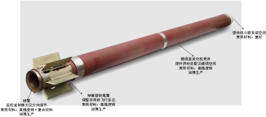
燃烧室发动机壳体及喷管壳体产品二
