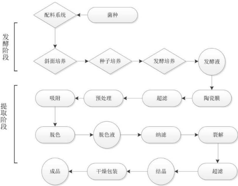
3、6-APA、青霉素 G 钾盐生产工艺流程图
