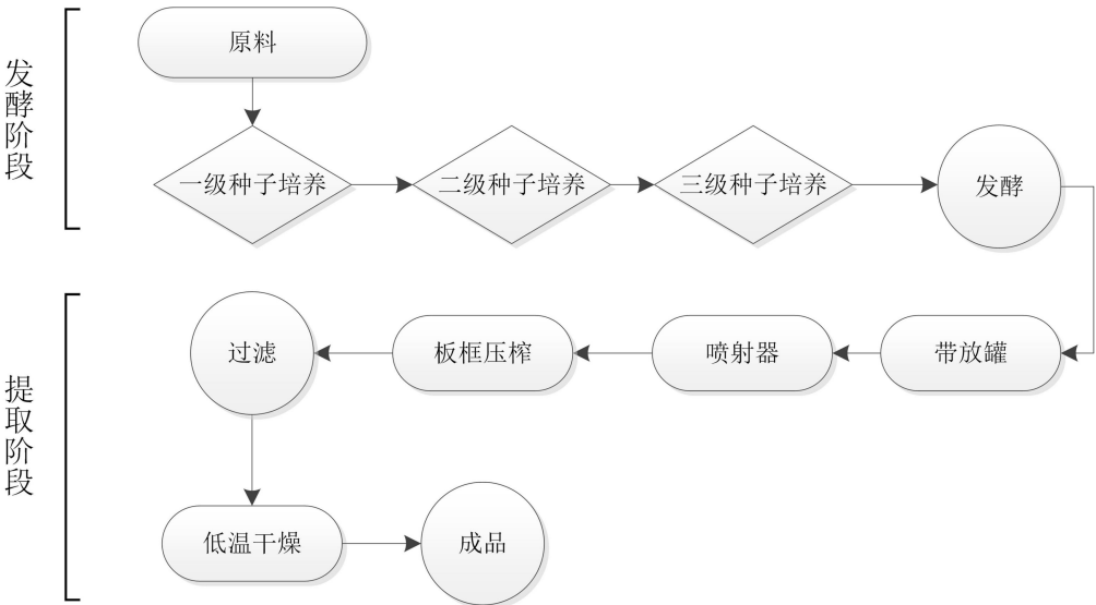
7、辅酶 Q10 菌丝体生产工艺流程图
