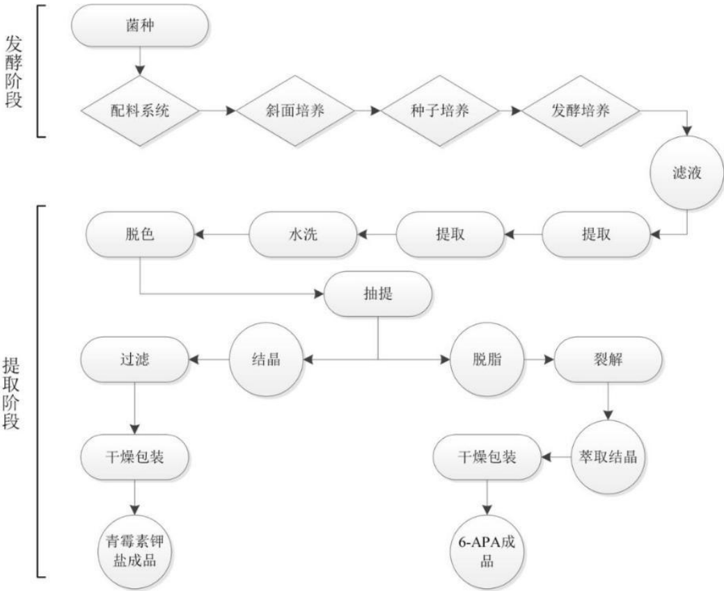
4、D-7ACA 生产工艺流程图
