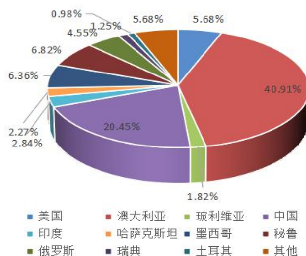
图 2-3 全球铅矿产资源储量分布占比图
