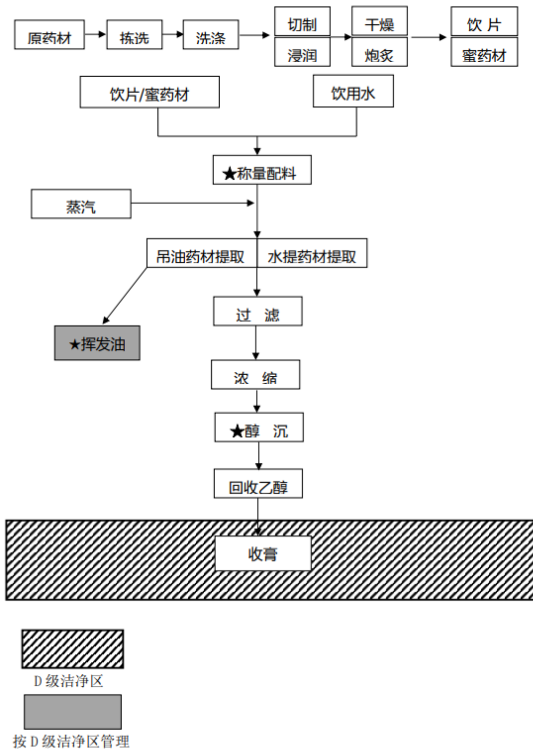
制剂车间生产工艺流程图：
