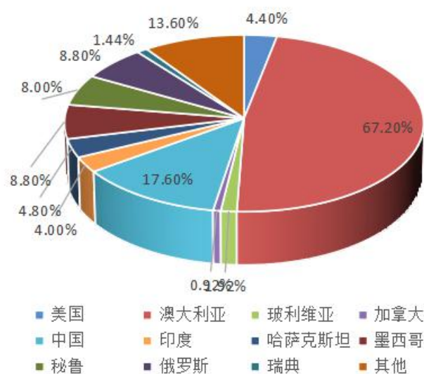
全球锌矿矿产资源储量分布占比数据来源：USGS
