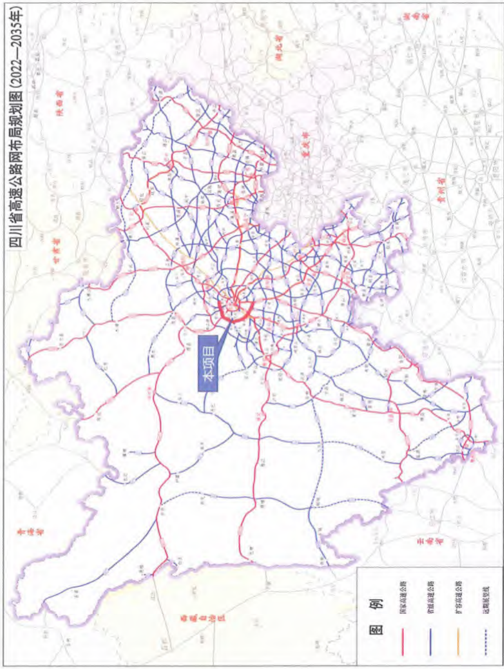
图1 成都第二绕城高速公路西段位置示意图
