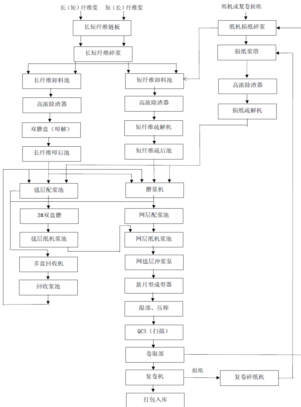
(4) 纸浆工艺流程图
