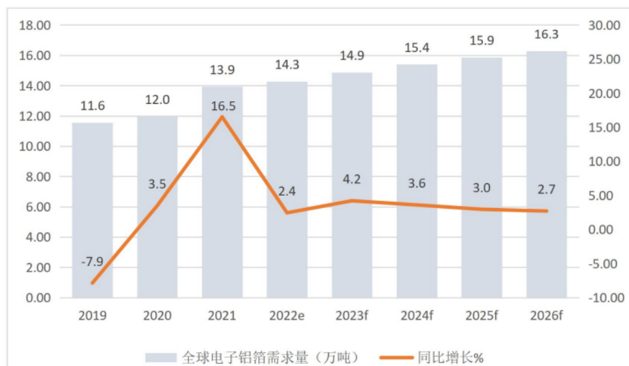
2019-2026 年全球电子铝箔需求量发展趋势与预测
