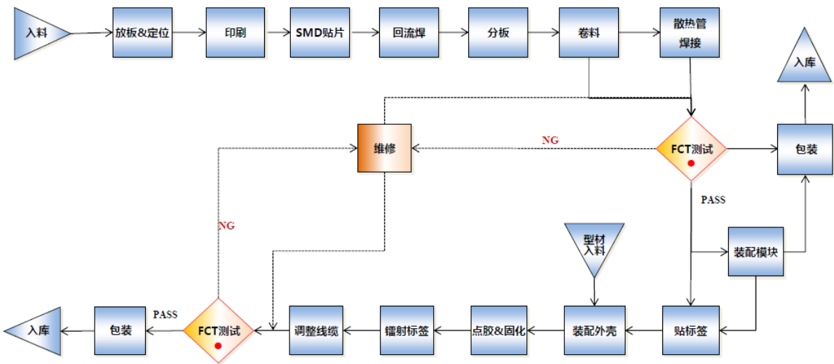
图：灯带标识产品生产工艺图
