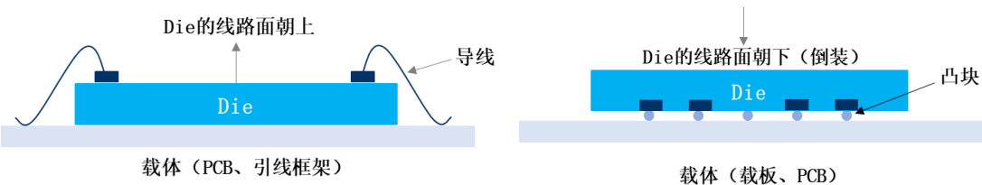
传统封装（打线）与先进封装（倒装）对比
