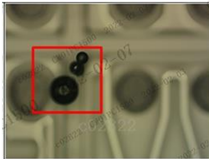
电子显微镜下的光阻气泡
