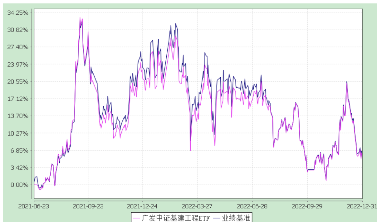
广发中证建设工程交易型开放式指数证券投资基金 份额累计净值增长率与业绩比较基准收益率的历史走势对比图 (2021年6月23日至2022年12月31日)
