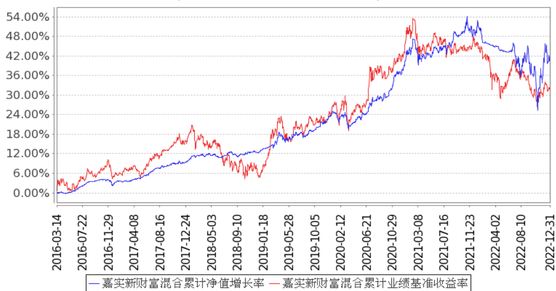
嘉实新财富混合累计净值增长率与同期业绩比较基准收益率的历史走势对比图 (2016年03月14日至2022年12月31日)
