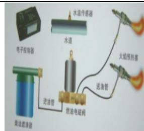
火焰预热装置
