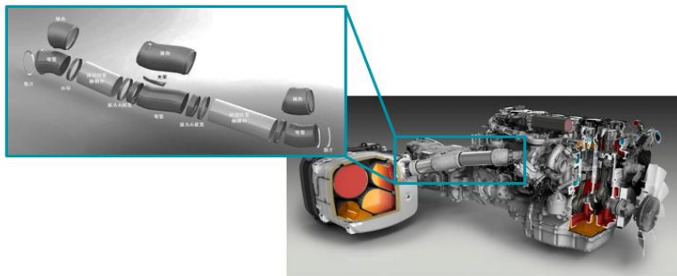
气密金属软管连接示意图
