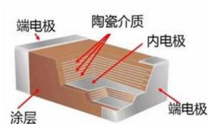
片式多层陶瓷电容器构造
