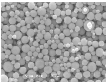
铜粉的电镜照片
