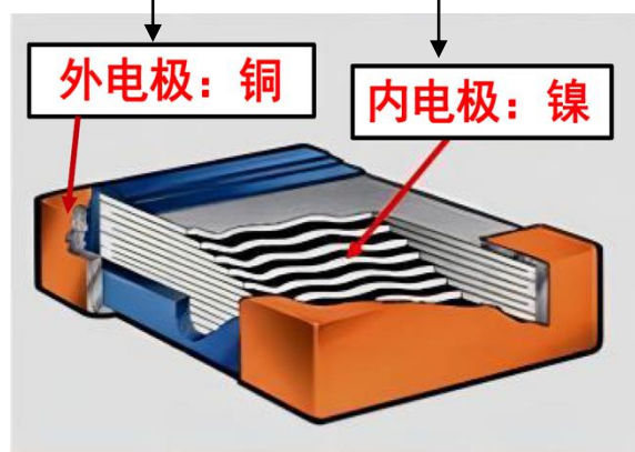
MLCC 剖面图
