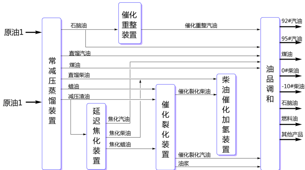
汽油生产流程图
